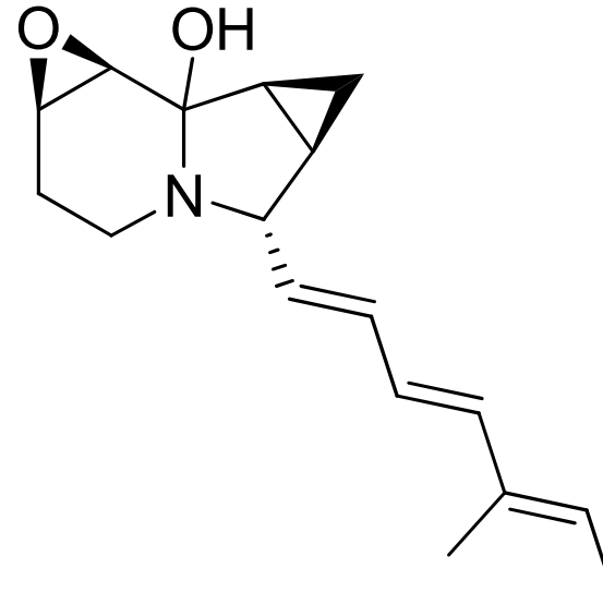
indolizomycin
