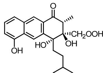
rishirilide B
