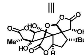
Ginkgolide B
