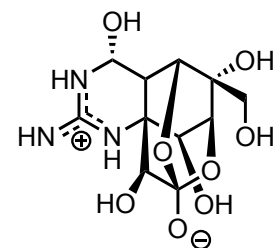
DL-tetrodotxin Kishi JACS 1972 , 94 , 9217.
