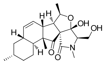
(-)-fusarisetin A
